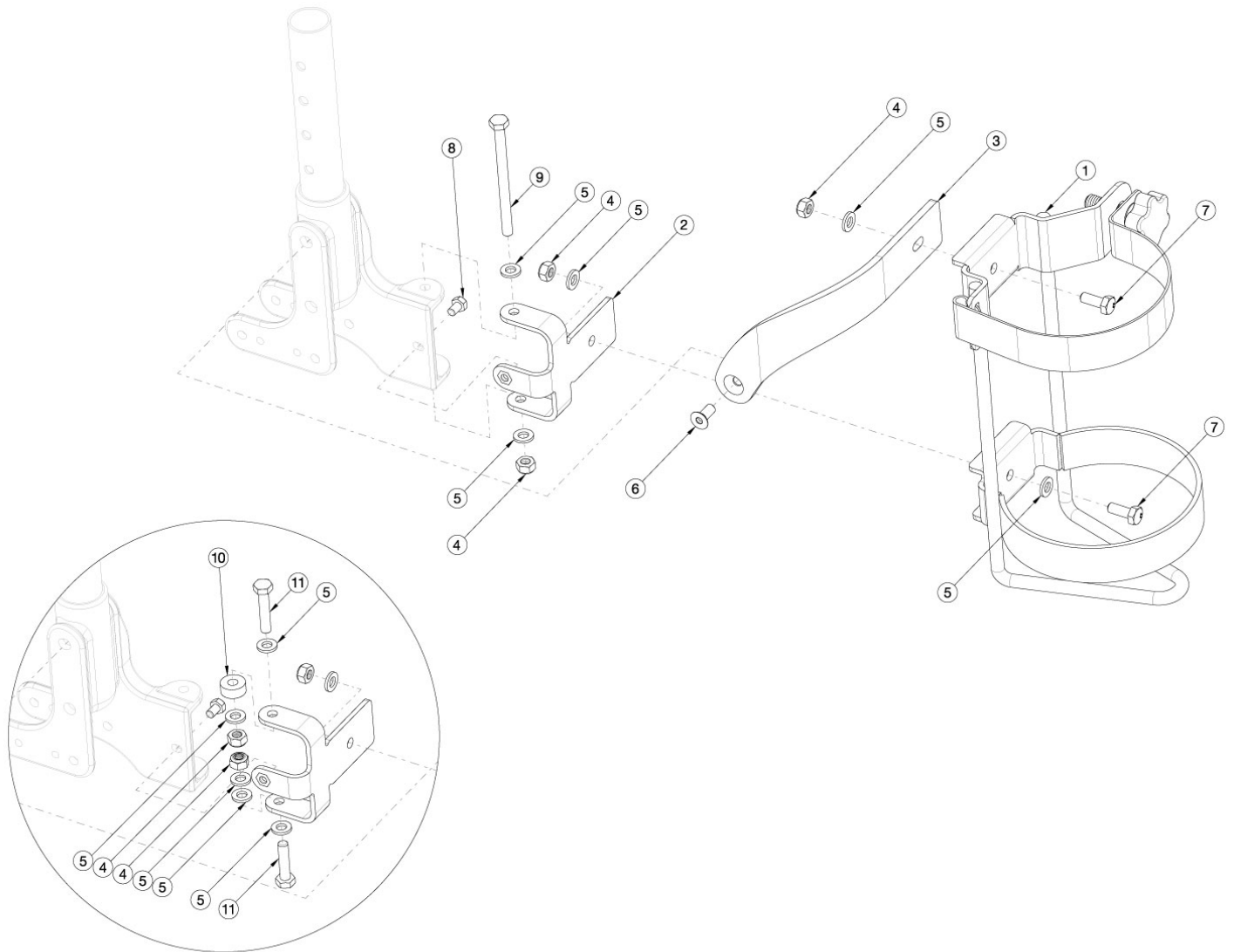
Rigid Frame Hardware
